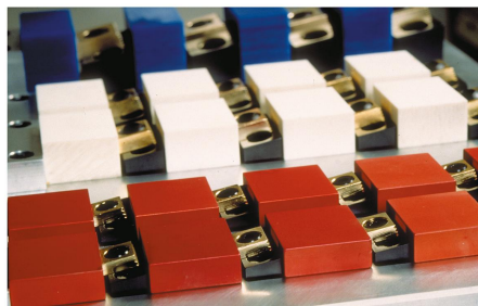
Пример применения многоместного зажима с комбинированными прижимными клещами
