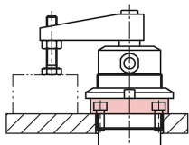
Pomocí závitové příruby a matice do drážky.
