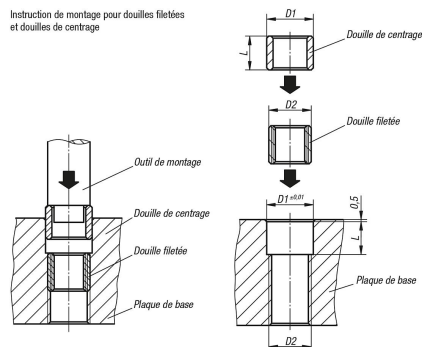
Instruction de montage pour douilles filetées et douilles de centrage
