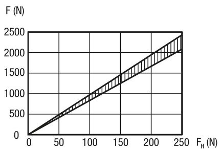
Diagramme des efforts
