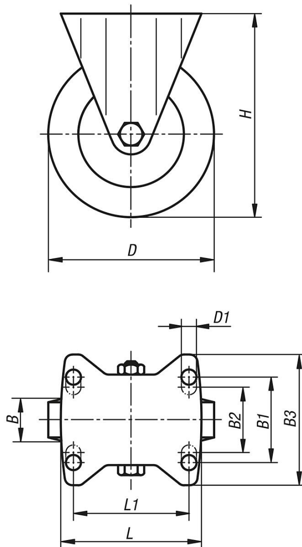
고정 캐스터
