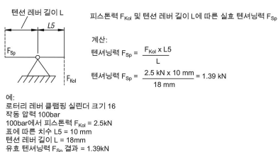
유압 로터리 레버 클램프의 유효한 텐션링력 계산:
