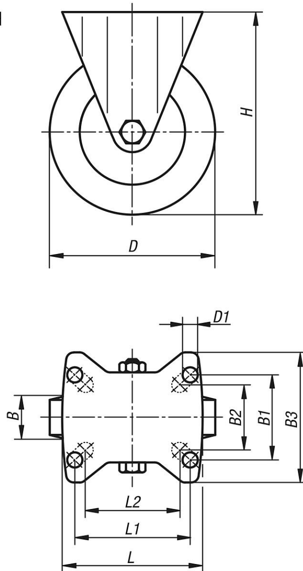
고정 캐스터
