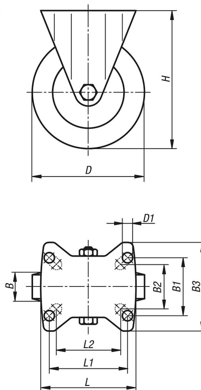
고정 캐스터
