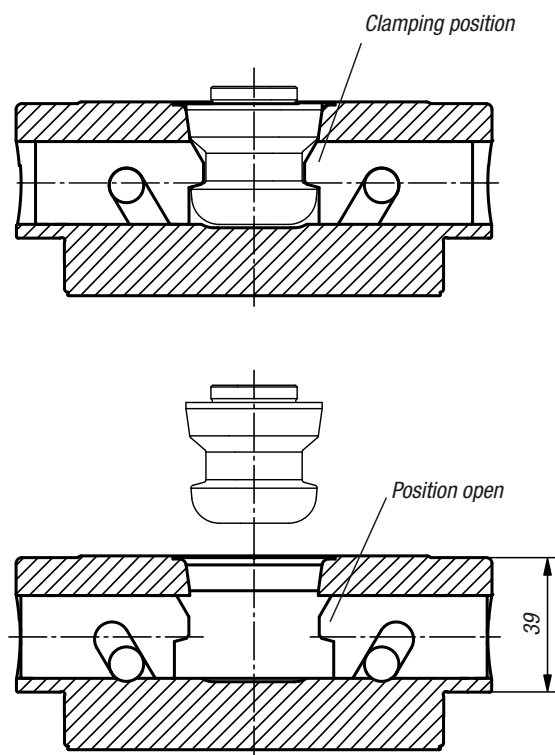
UNILOCK clamping module ESM 138-C UNILOCK clamping module ESM 176 UNILOCK clamping module EFM138
