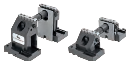
3-Achs-Spanner 5-Achs-Spanner
