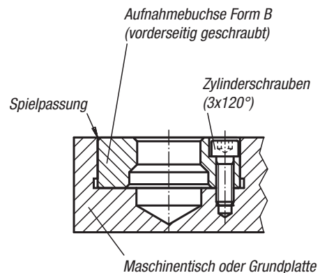
Alternativer Einbau
