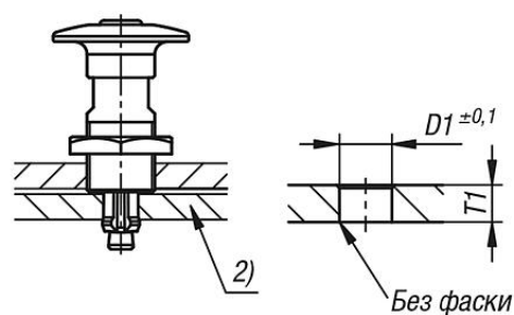
Крепежное отверстие в плите основания:
