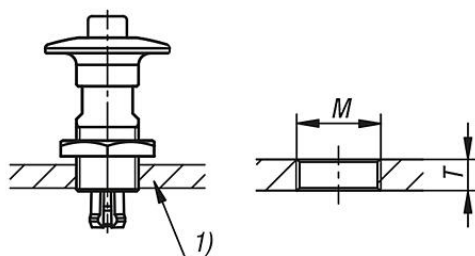
Крепежное отверстие в сопрягаемой плите:
