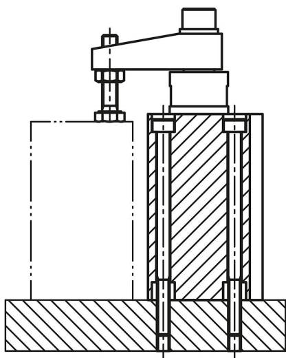
Пример монтажа:
