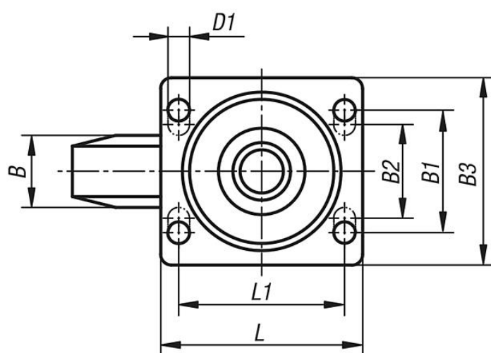
Подшипниковый узел поворотного венца:
