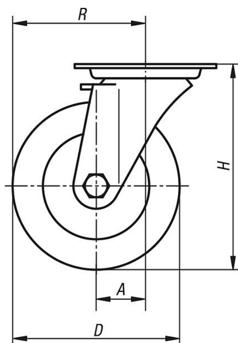
Поворотный ролик
