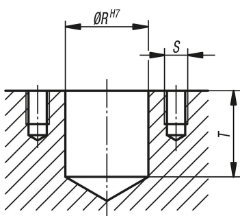
Dimensões do furo de alojamento
