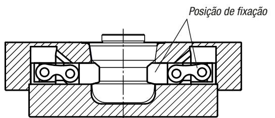
Módulo de fixação UNILOCK ERGO 138
